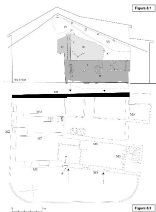
Relevé du mur mitoyen avec le quai d'Hermance 10 (côté quai d'Hermance 10)
